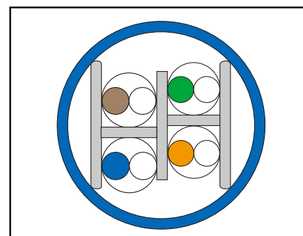
10GX 系列线缆的 RoundFlex 设计
