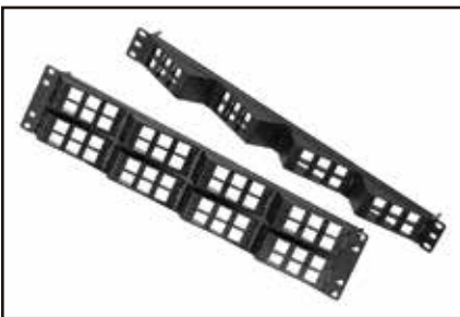
KeyConnect AngleFlex 配线架（空架）
