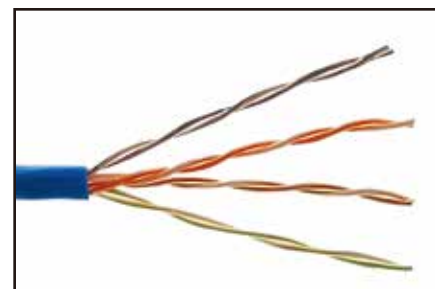
DataTwist 6阻燃通信线缆
