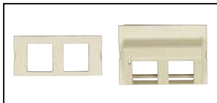
KeyConnect 模块用 MediaFlex 插件：AX102410，暗装插座，2 口，杏仁色和 AX102412，斜面，2 口，杏仁色
